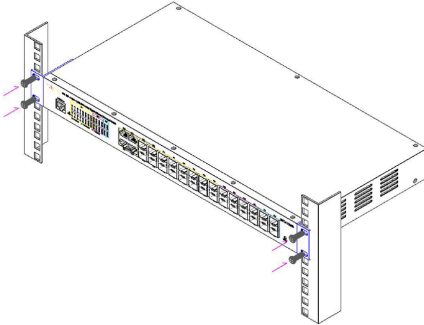
SFC4100AB Rack Mount 장착 모습
