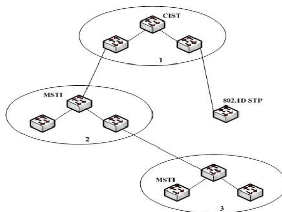
그림 2.1 MSTP 토폴로지
