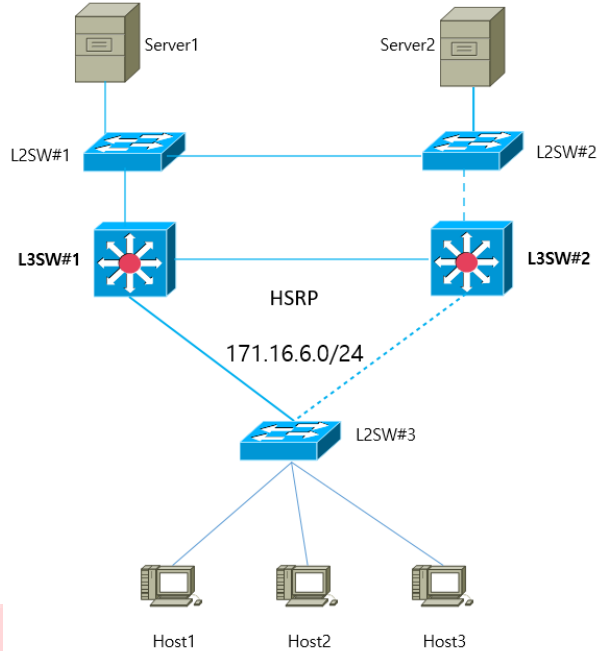
그림 2 - 1 HSRP 구성
