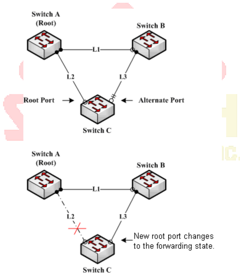
그림 1.3 Uplinkfast
