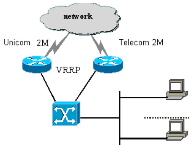
그림 3 - 1 VRRP 애플리케이션
