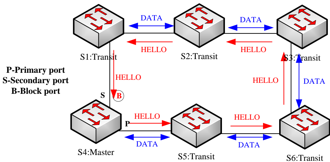
그림 3 폴링
