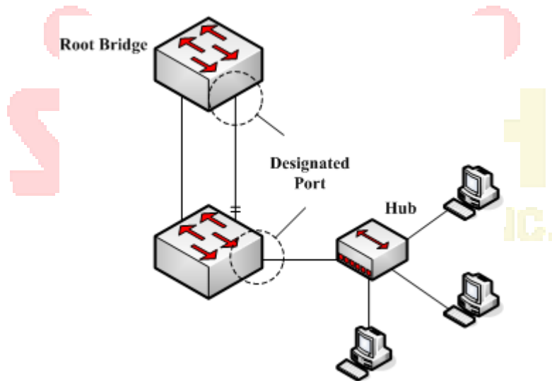
그림 2.4 지정된 포트
