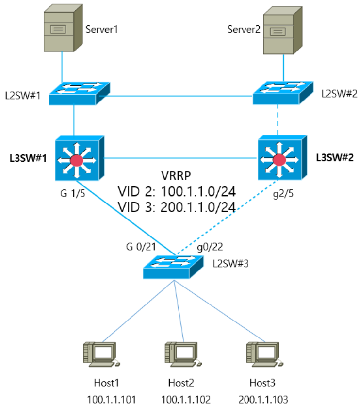
그림 3 - 2 단순 VRRP 애플리케이션 토폴로지
