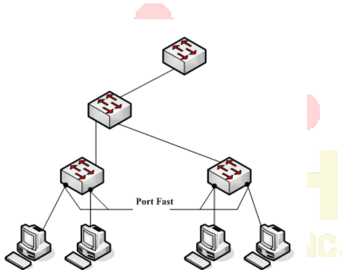
그림 1.1 Port Fast
