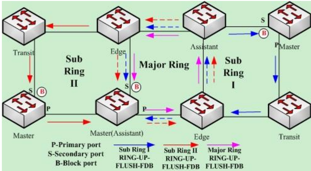
그림 15 링 복구
