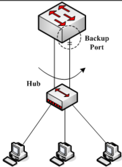
그림 2.5 백업 포트
