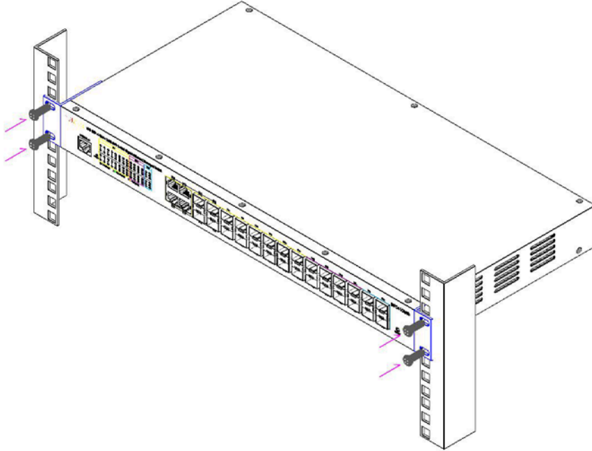
SFC6428AB Rack Mount 장착 모습
