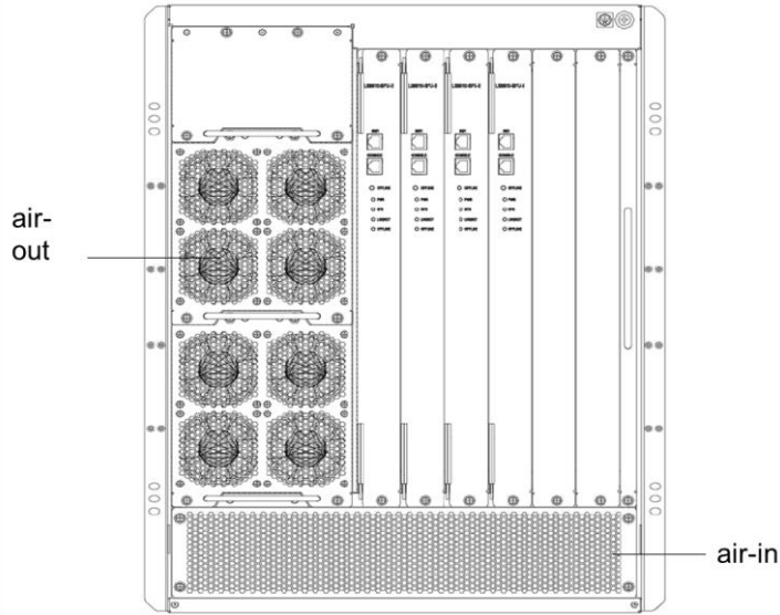
그림 2-2 SFC6510 제품군의 팬 흡기 배기 구조
