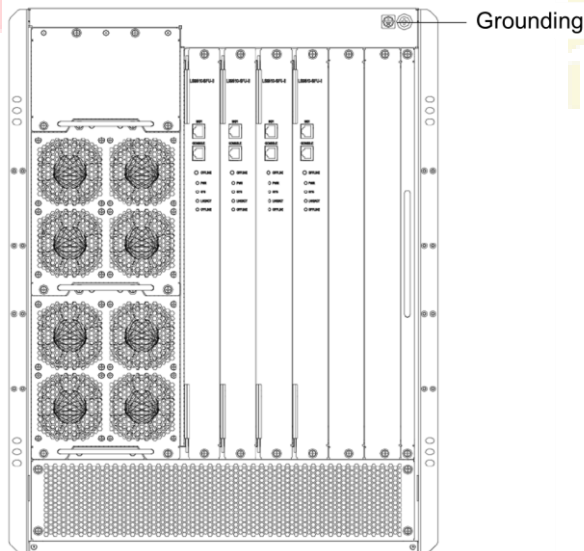
그림 2-3 SFC6510 접지 연결구 도면
