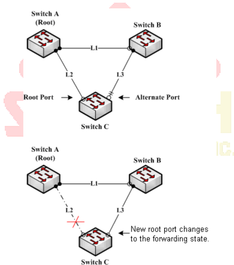
그림 1.3 Uplinkfast
