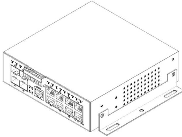
SFC8000G Wall Mount 브라켓 장착 모습
