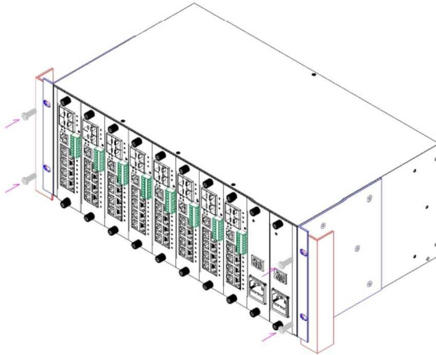
SFC8000G-4U Rack Mount 장착 모습
